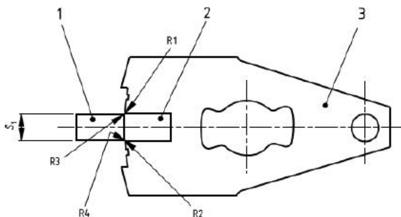
Рисунок В.2 - Схематическое представление радиусов скруглений на входе кодового канала и передней стороне стопорного элемента
