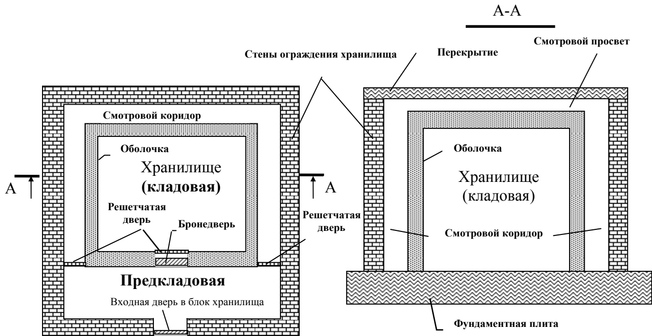
Рис. 7.3 Схематичное устройство хранилища ценностей
